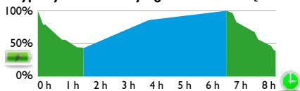
Typowy dzień roboczy 8 godz. z ładowarką e5
