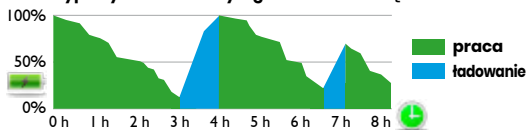
Typowy dzień roboczy 8 godz. z ładowarką e6
